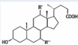
Bile acid
